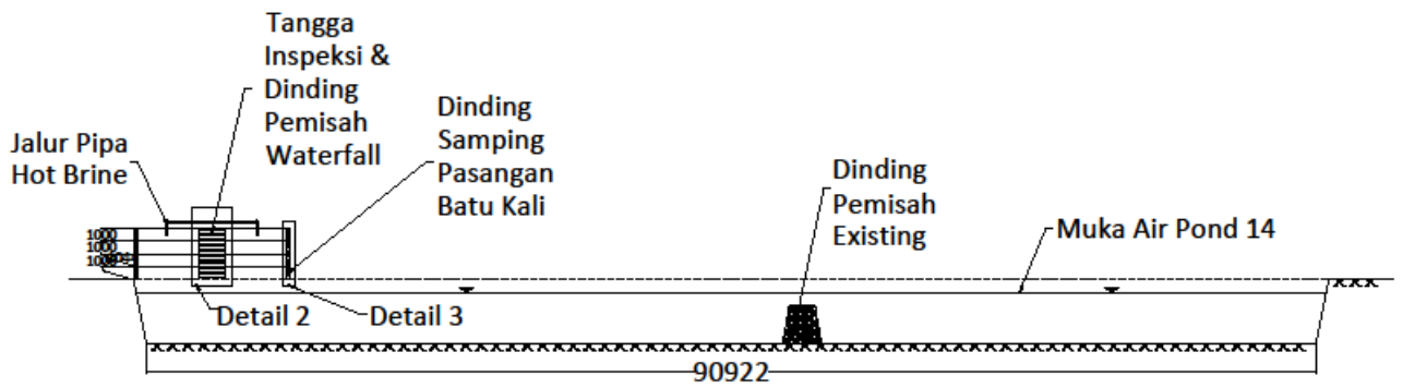
POTONGAN B SKALA NTS
