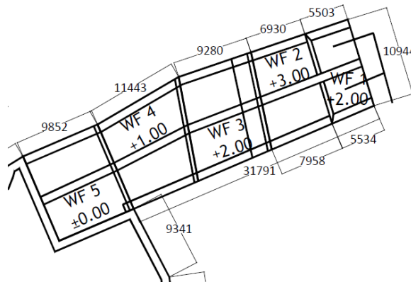
Gambar Rencana Sekat Pemisah Pond 14 (tampak atas)
