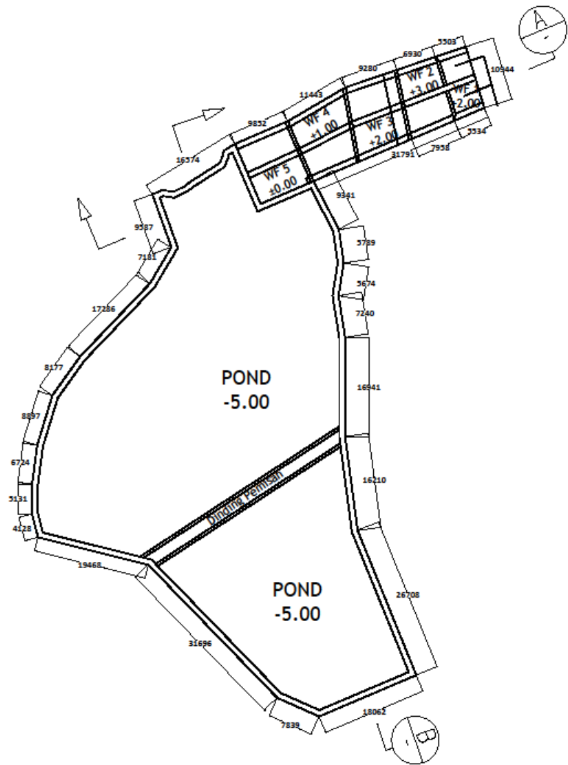
DENAH RENCANA PEKERJAAN POND & WATERFALL PAD 14 SKALA NTS
