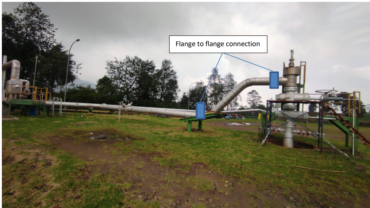
Gambar 1. Kondisi Sumur PPL-05 dan rencana pemasangan koneksi flange to flange
